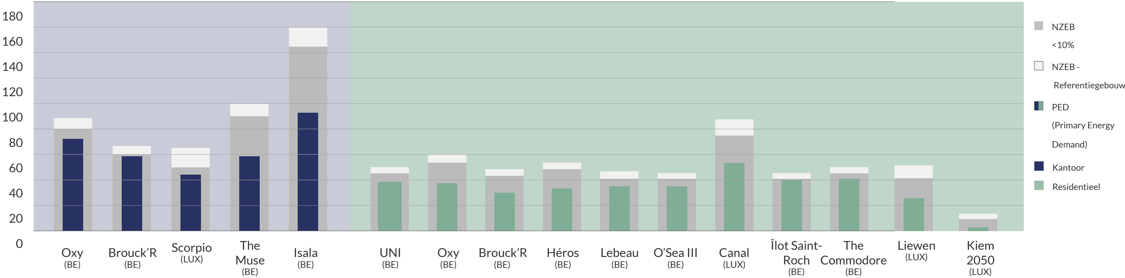
Primair energieverbruik (kWh/m 2 /jaar)
